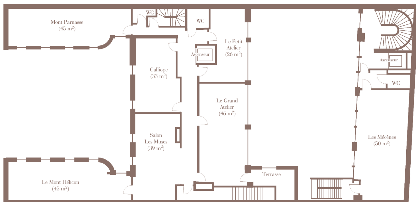
3 ème étage
