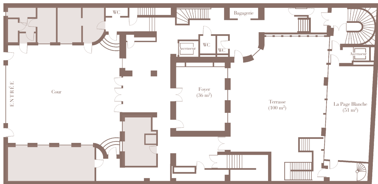
Rez-de-Chaussée
